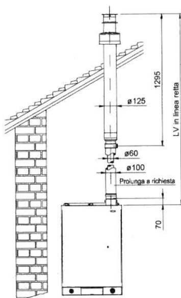
SOUOSÝ VERTIKÁLNÍ SYSTÉM ODTAHU SPALIN
