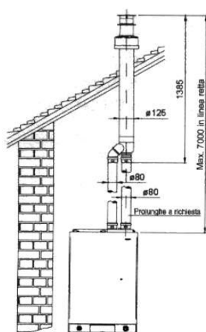
ROZDVOJENÉ POTRUBÍ SE SLUČOVAČEM A SOUOSÝM KOMÍNEM
