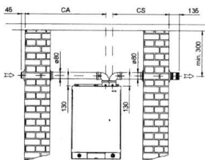
ROZDVOJENÝ ODTAH PŘES ZDIVO
