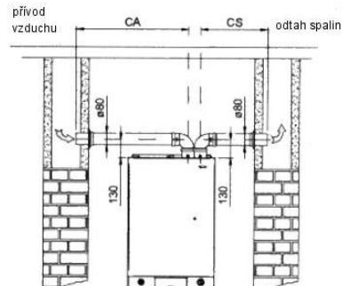
PŘÍVOD VZDUCHU POTRUBÍM ODTAH SPALIN DO KOMÍNA
