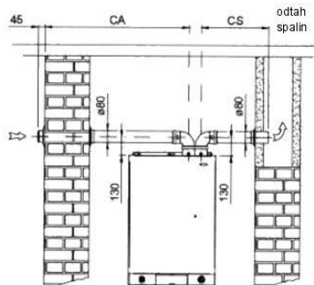
PŘÍVOD VZDUCHU PŘES ZDIVO ODTAH SPALIN DO KOMÍNA
