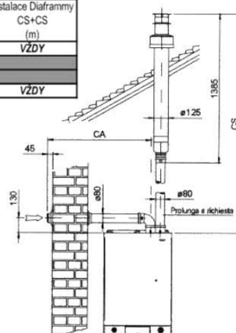
ROZDVOJENÉ POTRUBÍ S VERTIKÁLNÍM ODTAHEM SPALIN
